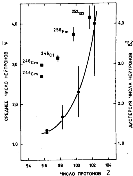
Рис. 4. Совокупность экспериментальных данных о \bar{\nu} (■) и \sigma_{\nu}^2 (●), полученных в настоящей работе (за исключением \bar{\nu} для ^{244}\text{Cm} ).
