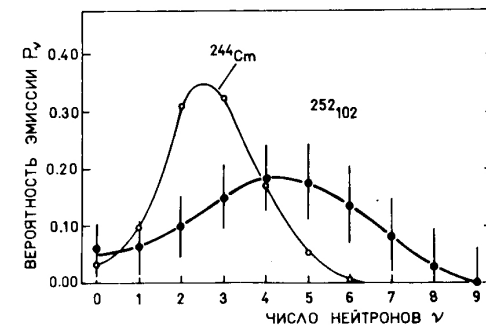
Рис. 3. Распределения множественности мгновенных нейтронов P_\nu в области кория-элемента 102, измеренные в настоящей работе.
